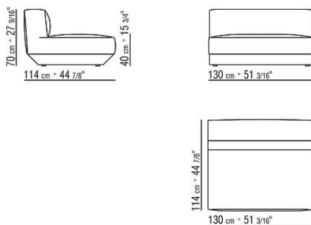
COD. 02D311 FIANCO SX
