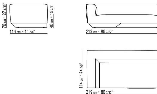
COD. 02D341 ELEMENTO TERMINALE SX
