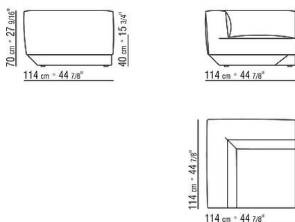
COD. 02D335 ANGOLO SX
