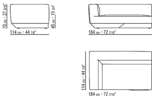
COD. 02D339 ANGOLO SX
