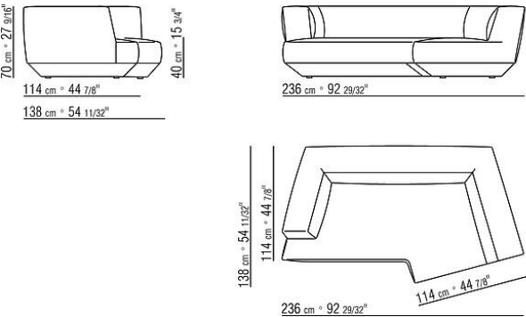
COD. 02D377 DIVANO / ANGOLO A 6 LATI SX
