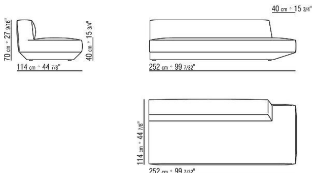
COD. 02D345 ELEMENTO TERMINALE SX
