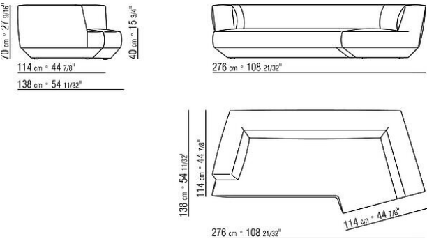
COD. 02D379 DIVANO / ANGOLO A 6 LATI SX
