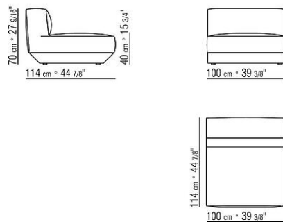
COD. 02D309 ELEMENTO
