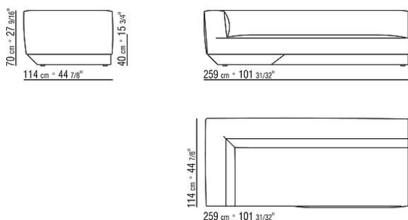
COD. 02D343 ELEMENTO TERMINALE SX
