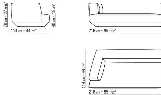
COD. 02D321 FIANCO TERMINALE SX
