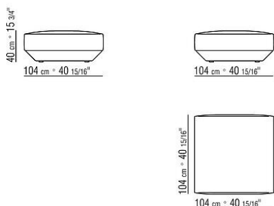
COD. 02D352 POUF CENTRALE
