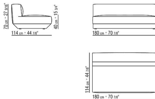
COD. 02D313 FIANCO SX
