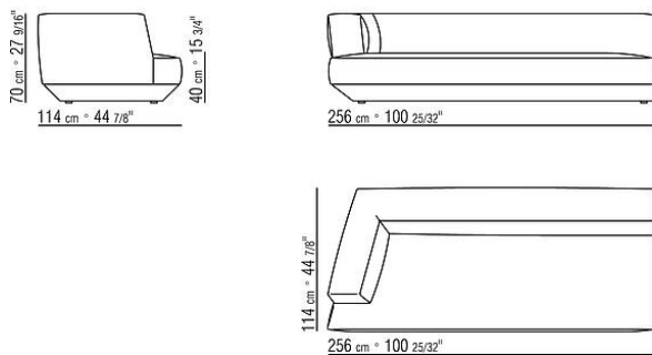
COD. 02D319 FIANCO SX
