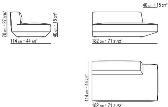
COD. 02D341 ELEMENTO TERMINALE SX
