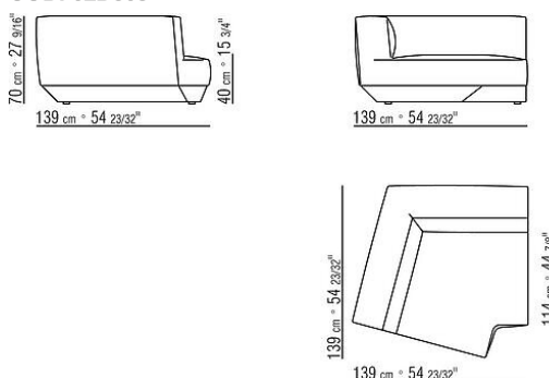
COD. 02D368 ANGOLO A 6 LATI
