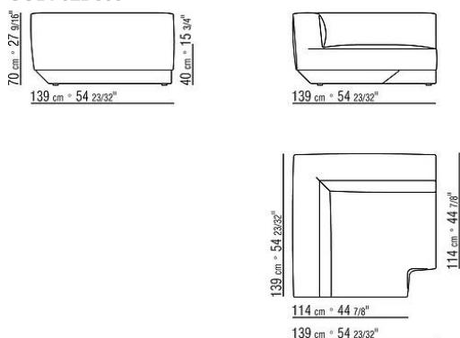
COD. 02D366 ANGOLO
