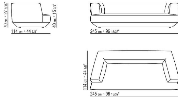
COD. 02D307 ELEMENTO
