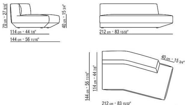
COD. 02D347 ELEMENTO TERMINALE A 6 LATI SX
